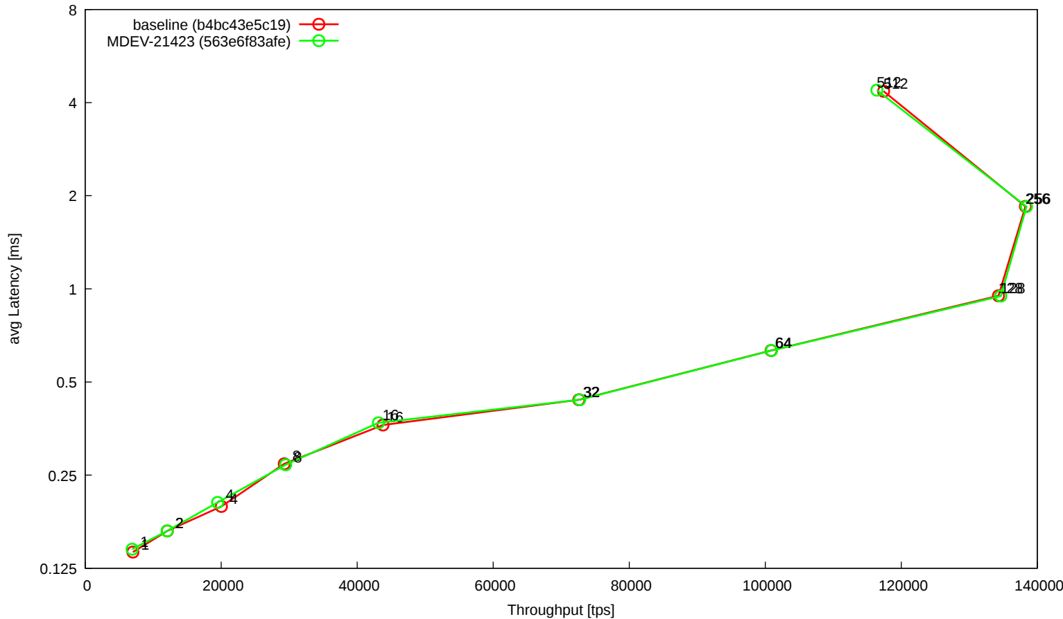
t_oltp_insert_innodb (@cheetah02)
