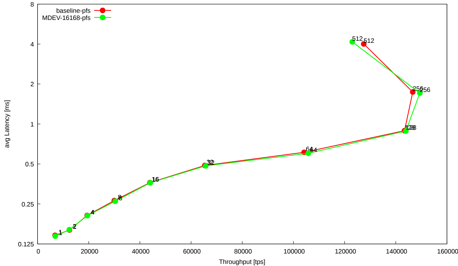
workload 't_oltp_insert_innodb'
