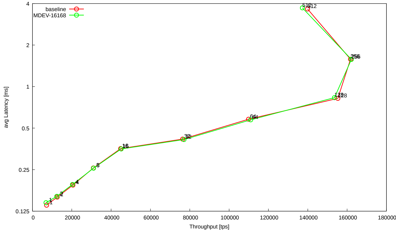
workload 't_oltp_insert_innodb'
