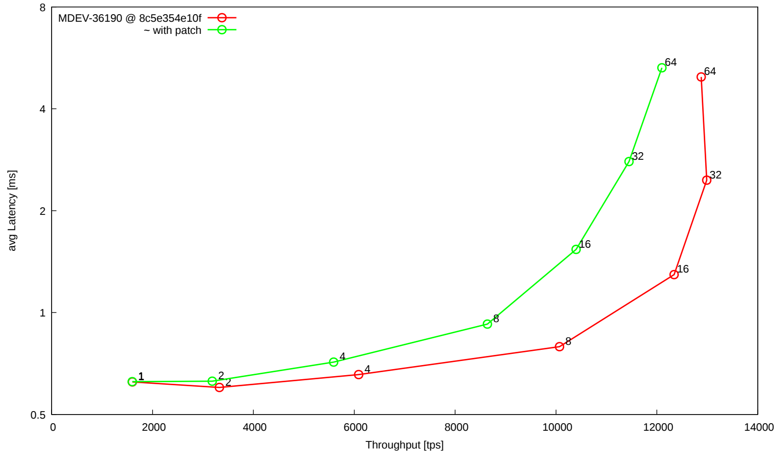
t_oltp_9010_innodb
