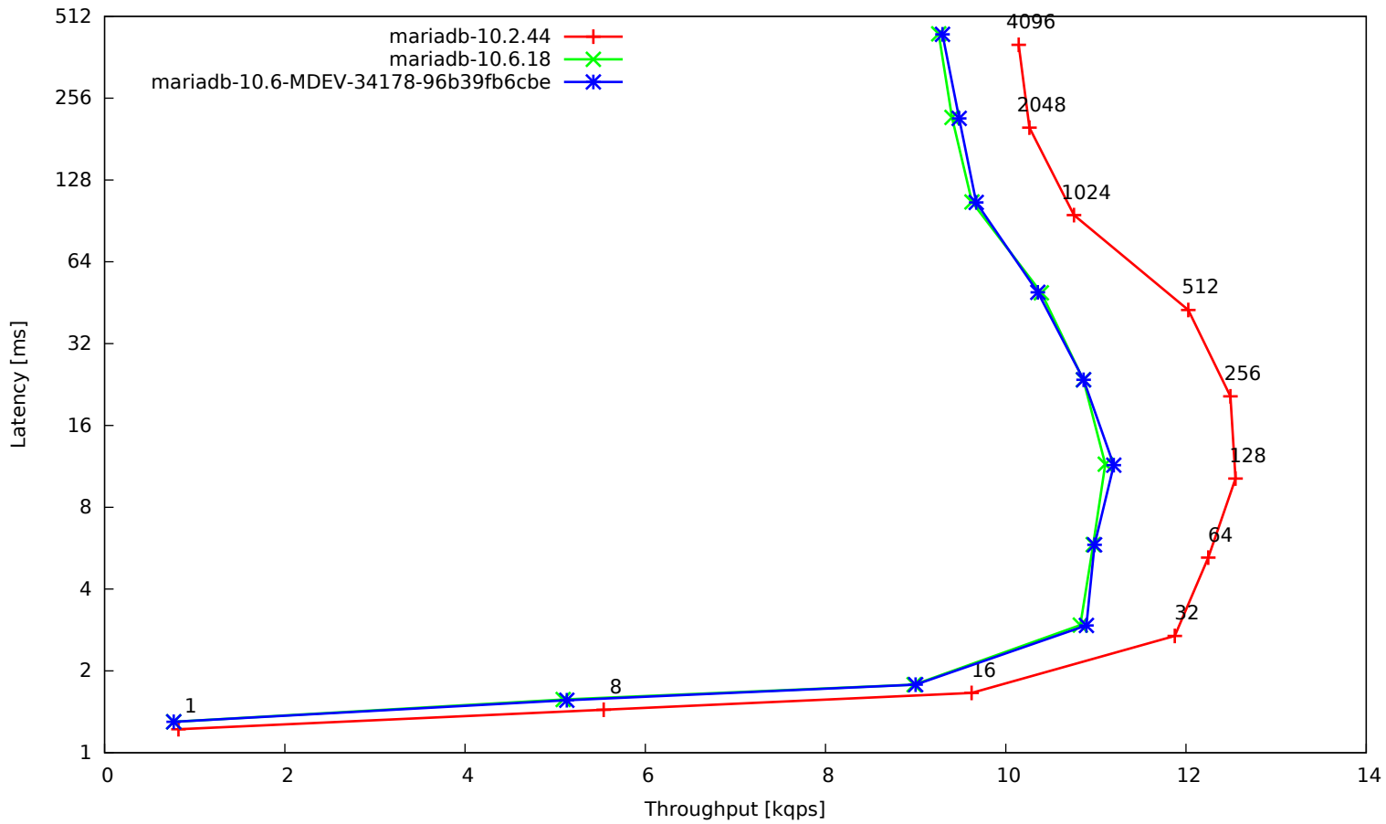
t_threadpool_on
