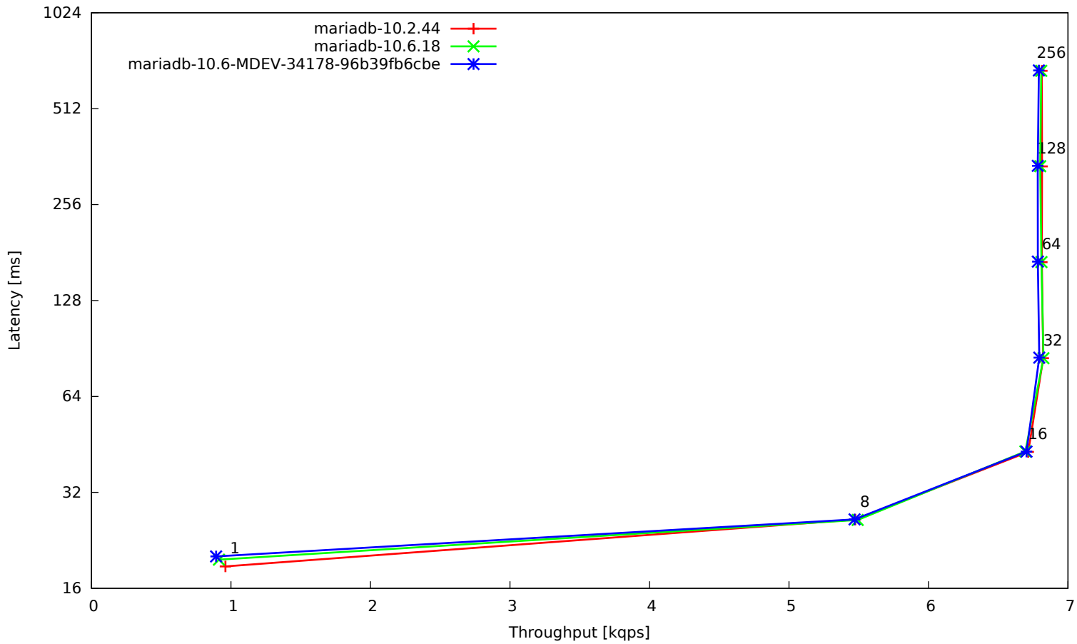
t_oltp-memory-multi
