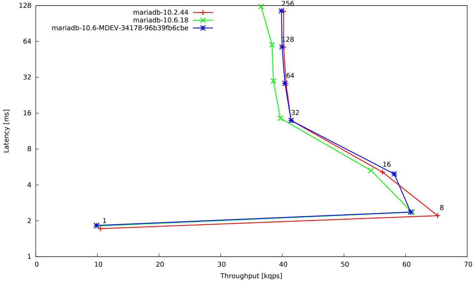
t_oltp-myisam-multi
