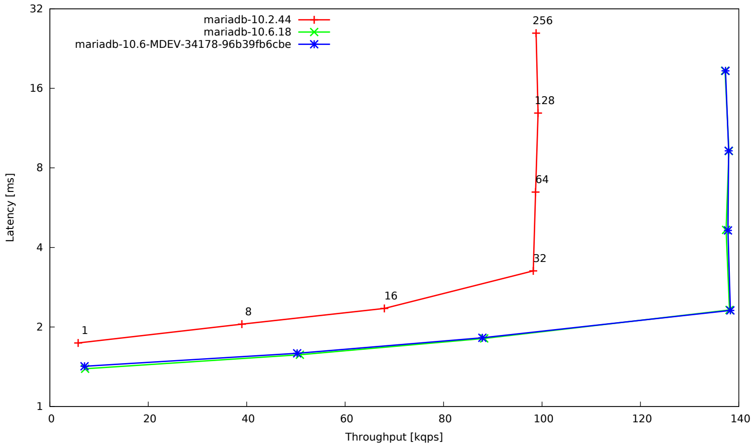
t_collate_distinct_range_utf8mb4_unicode
