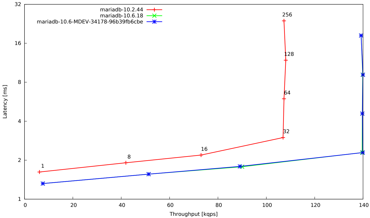
t_collate_distinct_range_utf8_unicode
