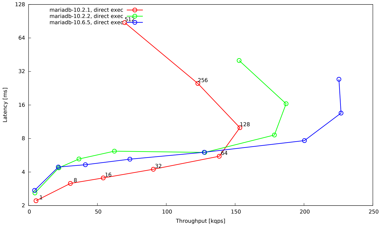
OLTP update indexed column (10 per TRX), 32 tables, 1 mio rows each, big BP, SSD
