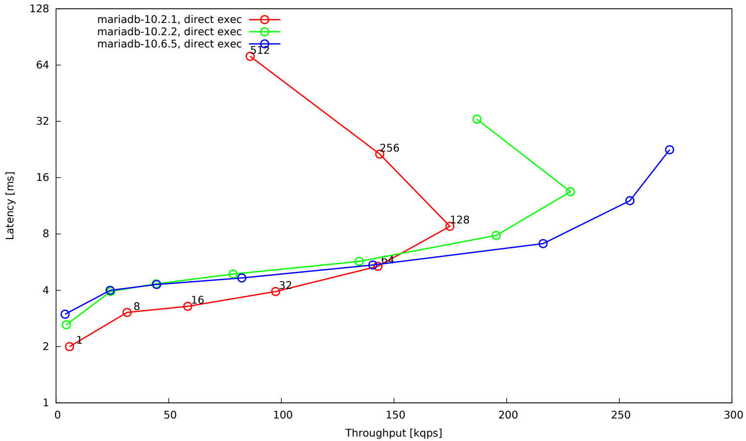
OLTP update unindexed column (10 per TRX), 32 tables, 1 mio rows each, big BP, SSD
