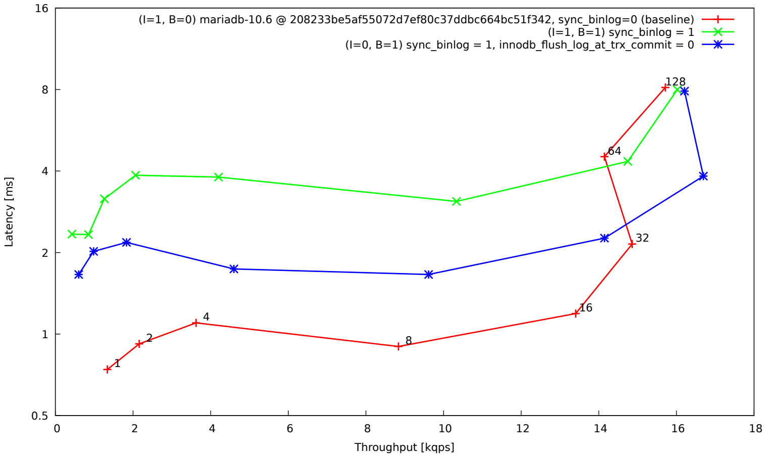
OLTP oltp_insert.lua default mix, 16 tables, 1 mio rows each, big BP, SSD
